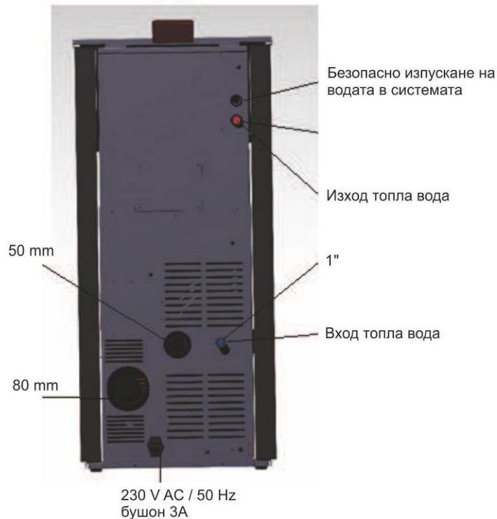
Фигура 3.11. Свързване на хидравличната система на камината.
